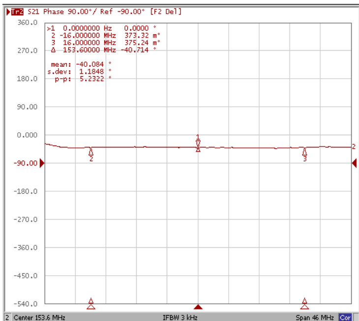
Phase ripple Fo±16.00MHz
