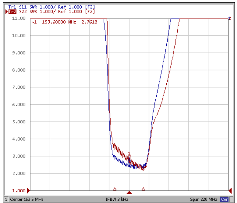
VSWR
