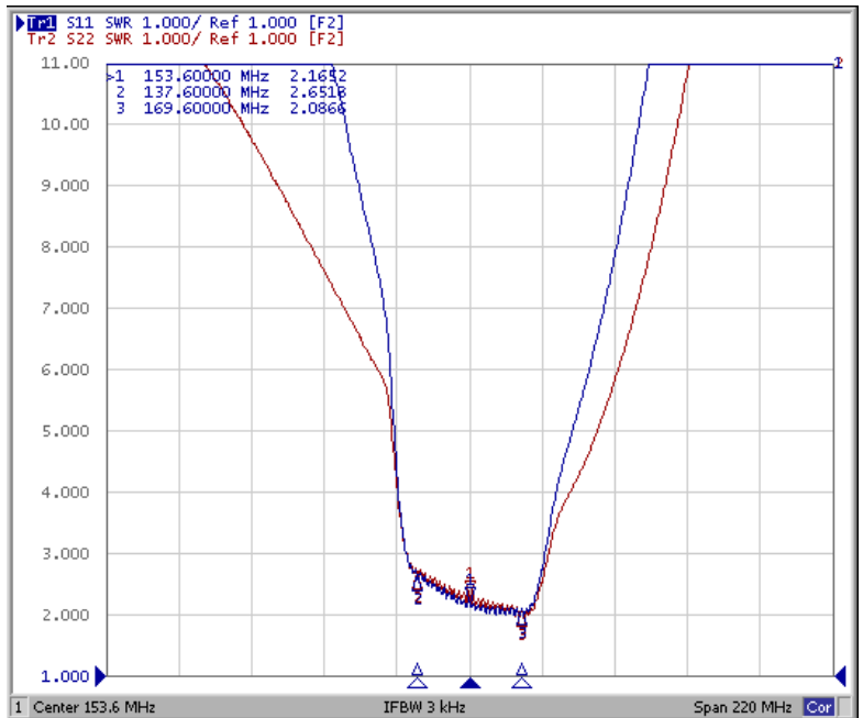
VSWR
